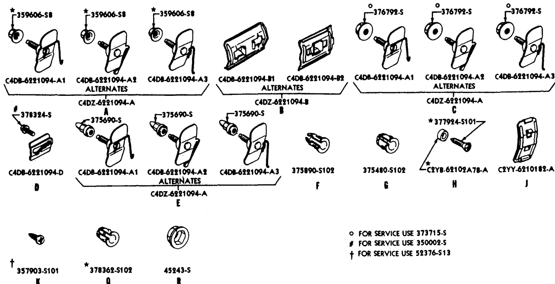
1964 FALCON FORDOR SEDAN - BODY TYPE X (54D)
